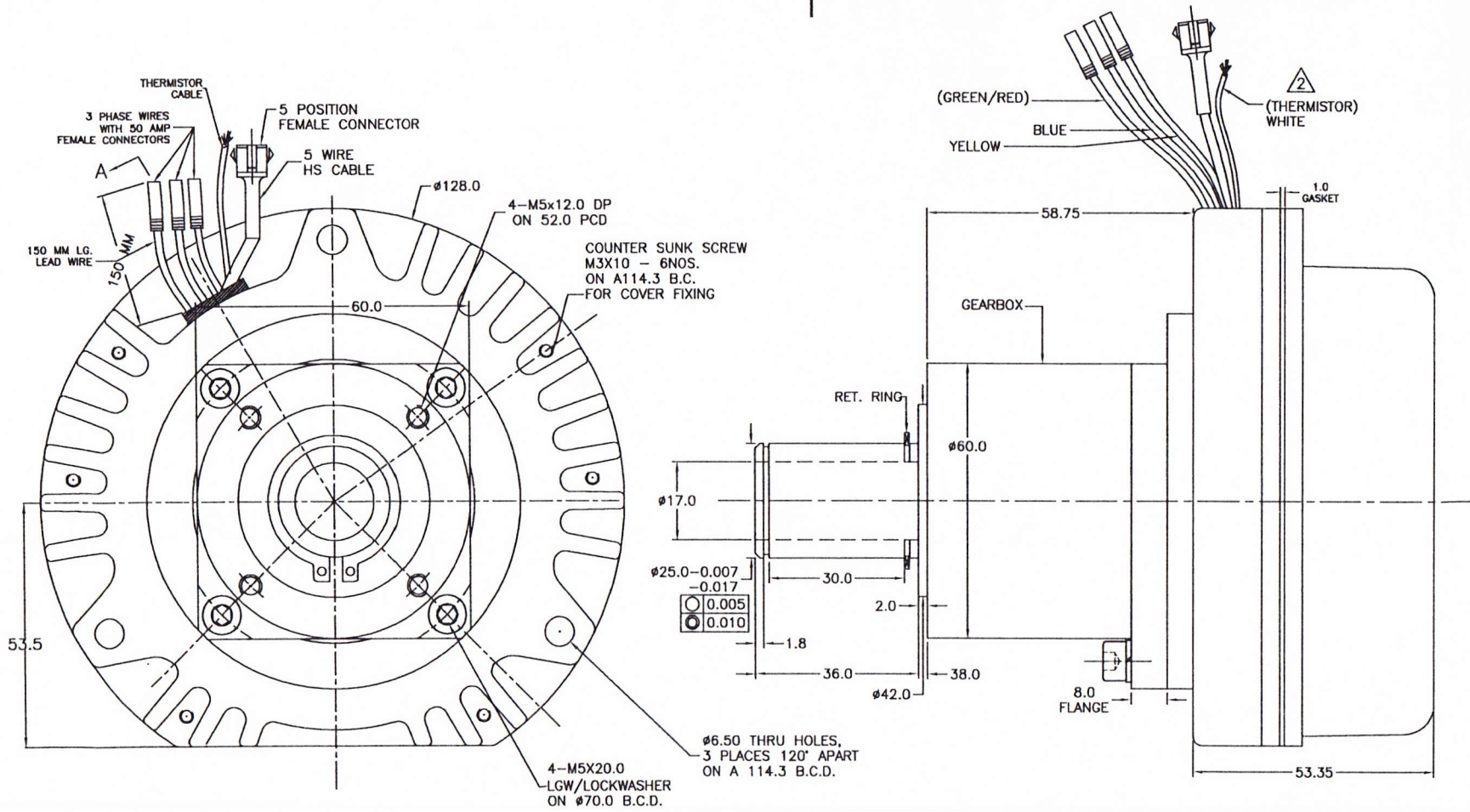
SECTION A-A
